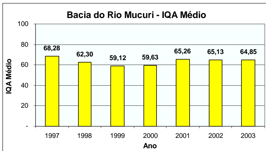
Figura 9.1: Evolução Temporal do IQA Médio na Bacia do Rio Mucuri.
