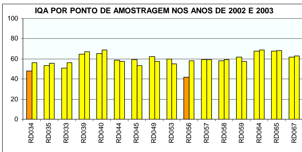
Figura 8.8: IQA médio dos anos 2002 e 2003, respectivamente, por estação de amostragem – UGRHs DO1 a DO5
