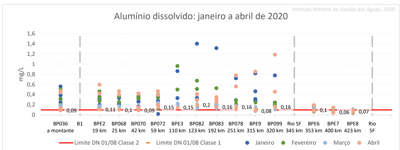
Figura 7: Resultados do monitoramento emergencial de alumínio dissolvido nos pontos de monitoramento do rio Paraopeba de janeiro a abril de 2020.
