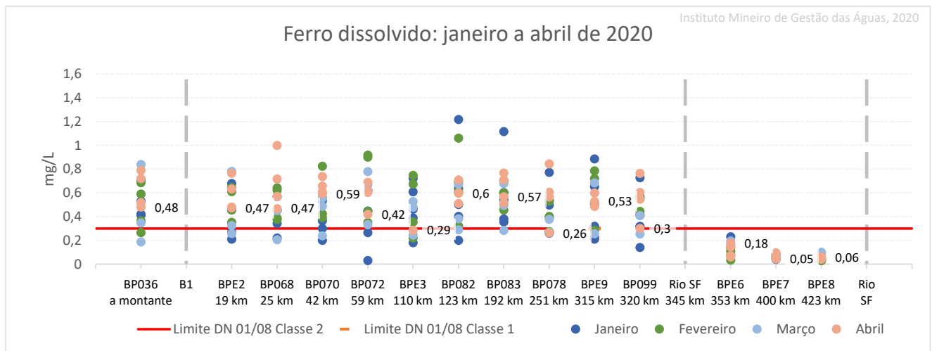
Figura 6: Resultados do monitoramento emergencial de ferro dissolvido nos pontos de monitoramento do rio Paraopeba de janeiro a abril de 2020.
