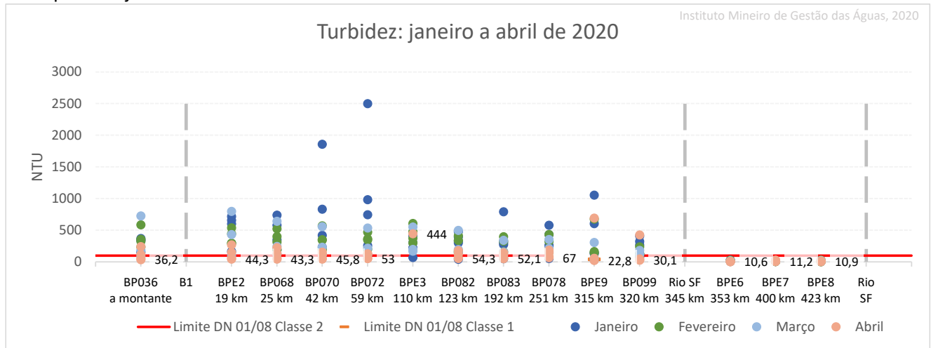
Figura 3: Resultados do monitoramento emergencial de turbidez nos pontos de monitoramento do rio Paraopeba de janeiro a abril de 2020.
