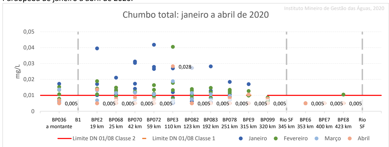
Figura 8: Resultados do monitoramento emergencial de chumbo total nos pontos de monitoramento do rio Paraopeba de janeiro a abril de 2020.
