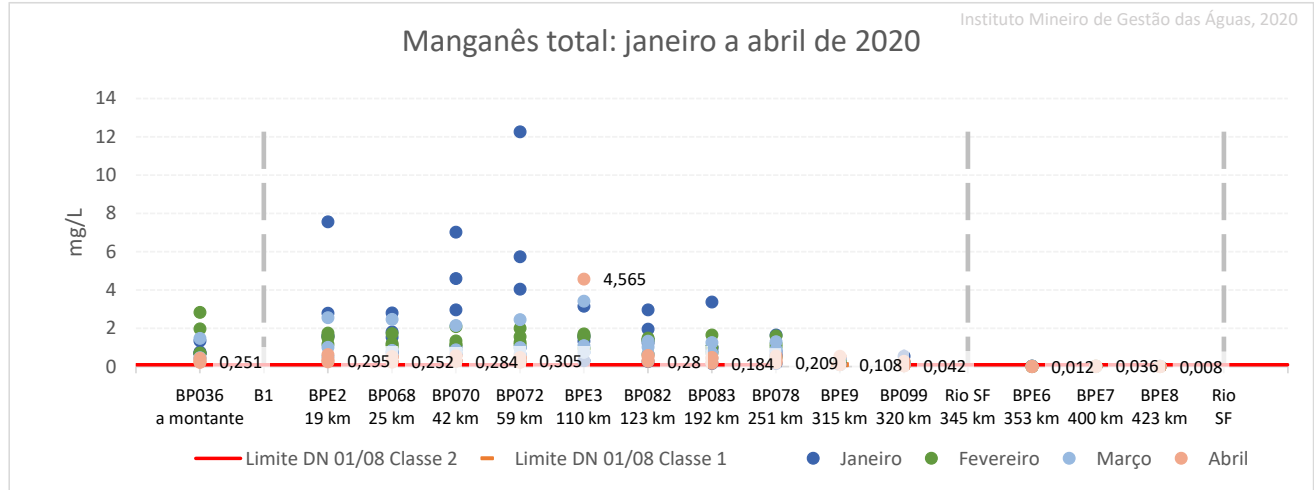
Figura 4: Resultados do monitoramento emergencial de manganês total nos pontos de monitoramento do rio Paraopeba de janeiro a abril de 2020.
