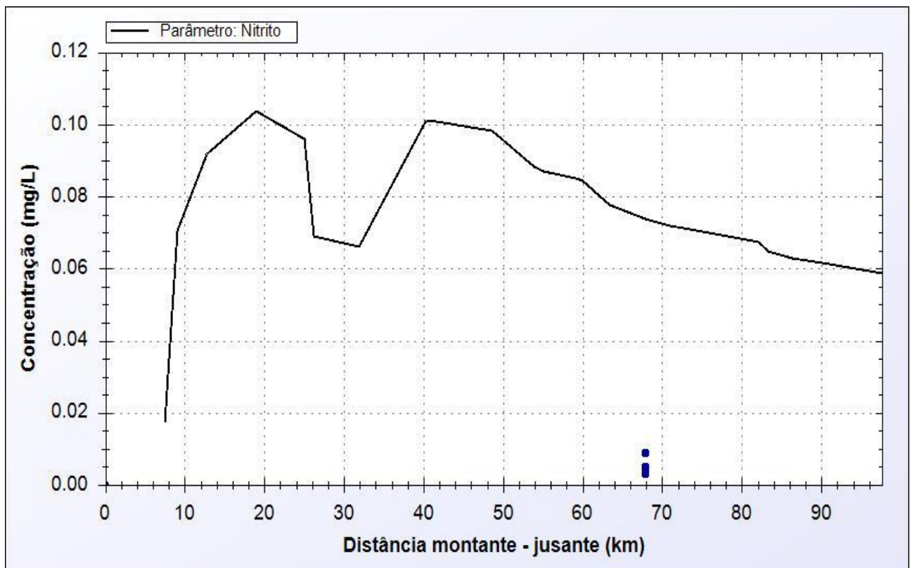
Figura 5.9 - Perfil de concentração ao longo do Rio Cricaré: nitrito.
