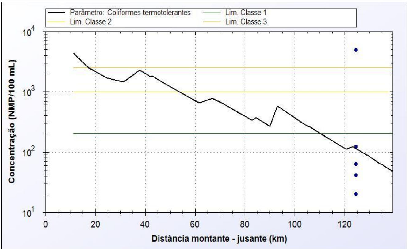
Figura 5.13 - Perfil de concentração ao longo do Rio Cotaxé: coliformes termotolerantes.
