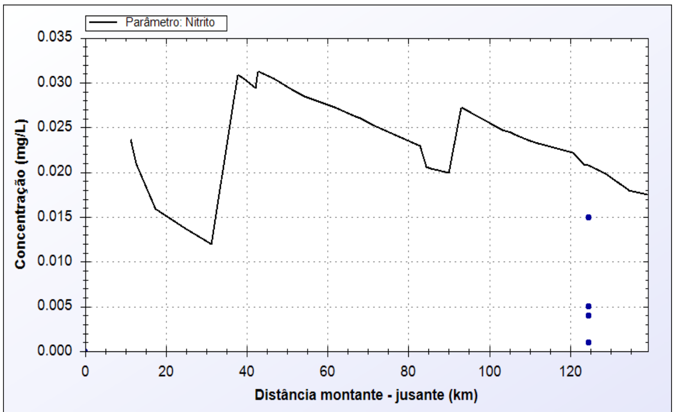
Figura 5.16 - Perfil de concentração ao longo do Rio Cotaxé: nitrito.
