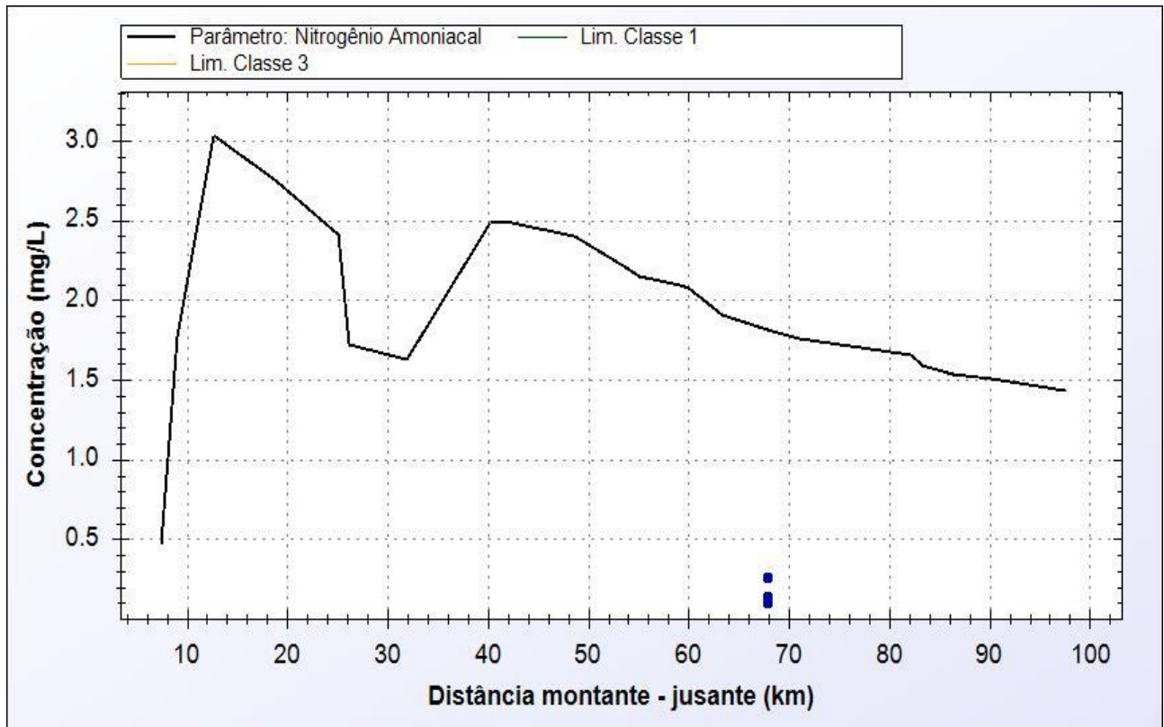
Figura 5.8 - Perfil de concentração ao longo do Rio Cricaré: nitrogênio amoniacal.
