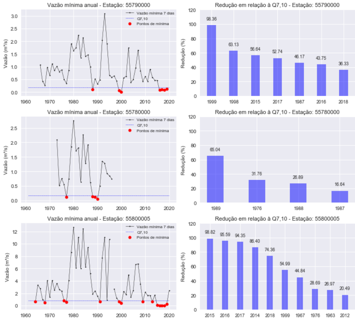
Figura 3.2 - Análise das séries de vazões mínimas anuais de sete dias de duração e comparativo com a Q_{7,10} nas estações fluviométricas da Bacia Hidrográfica do Rio São Mateus (Afluentes do Rio Cotaxé).
