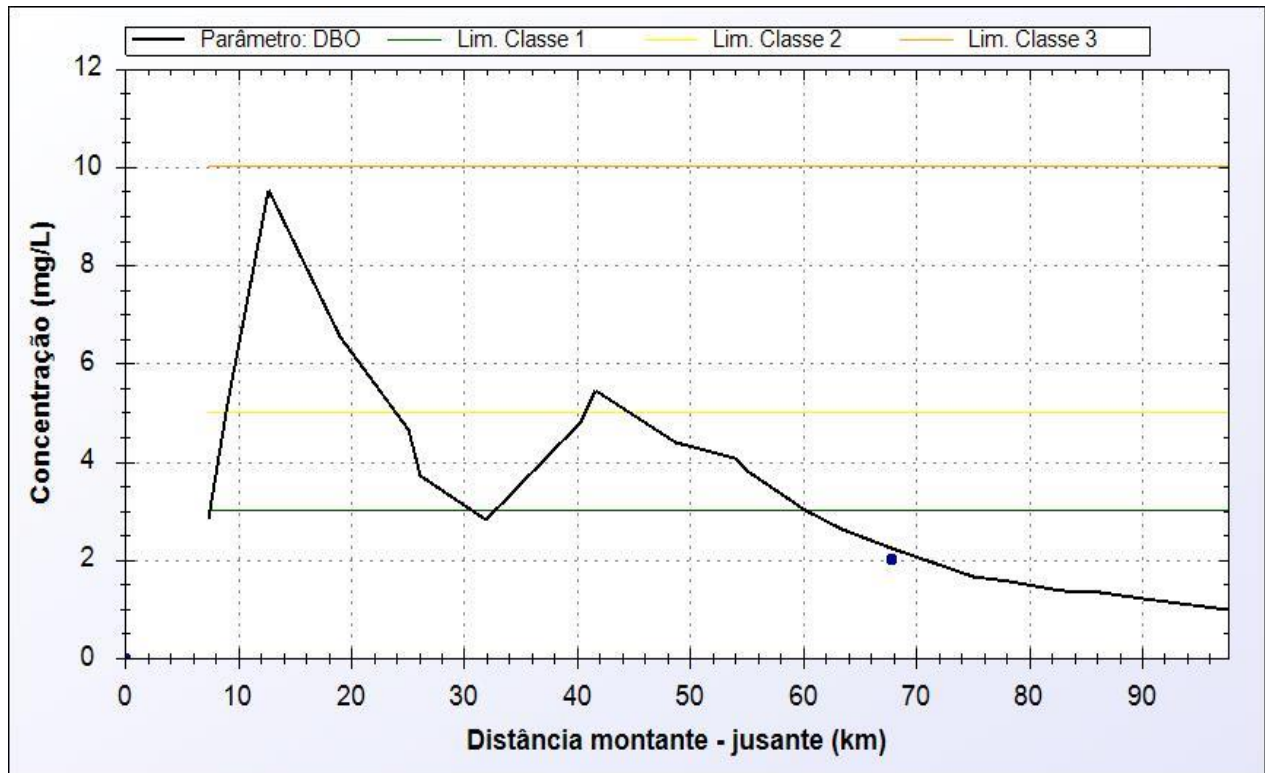
Figura 5.4 - Perfil de concentração ao longo do Rio Cricaré: DBO.
