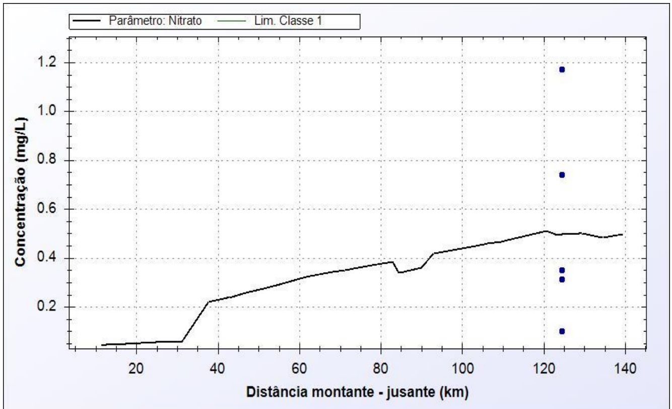
Figura 5.17 - Perfil de concentração ao longo do Rio Cotaxé: nitrato.
