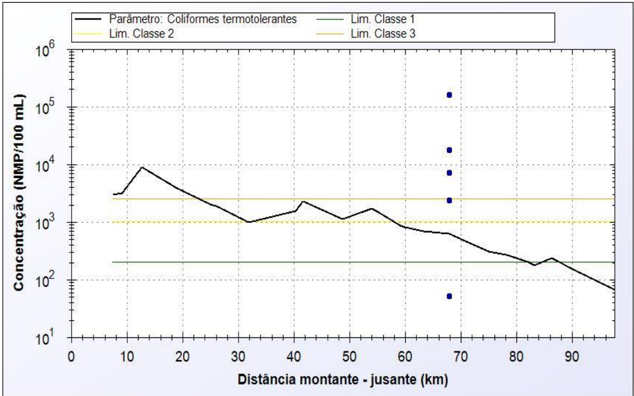
Figura 5.6 - Perfil de concentração ao longo do Rio Cricaré: coliformes termotolerantes.
