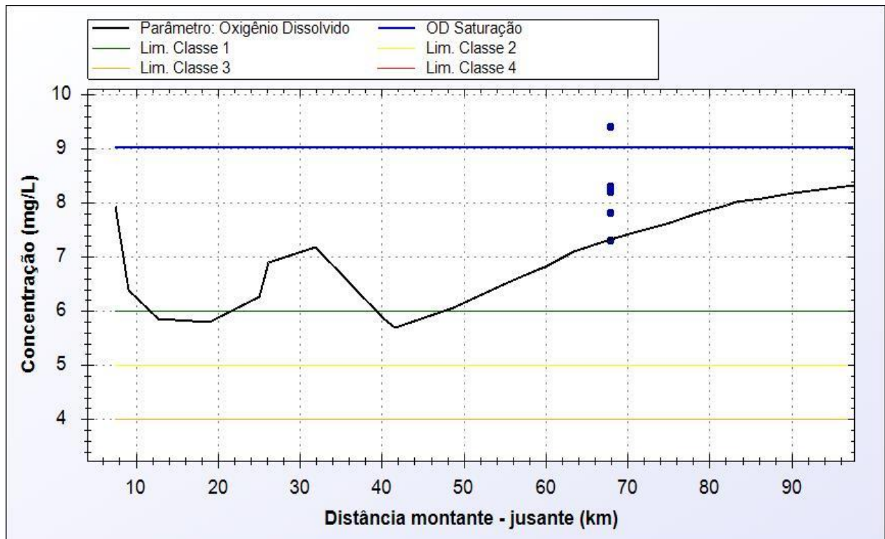
Figura 5.5 - Perfil de concentração ao longo do Rio Cricaré: OD.
