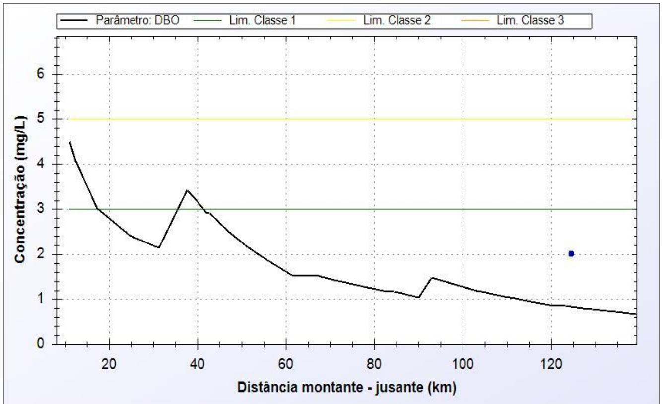
Figura 5.11 - Perfil de concentração ao longo do Rio Cotaxé: DBO.
