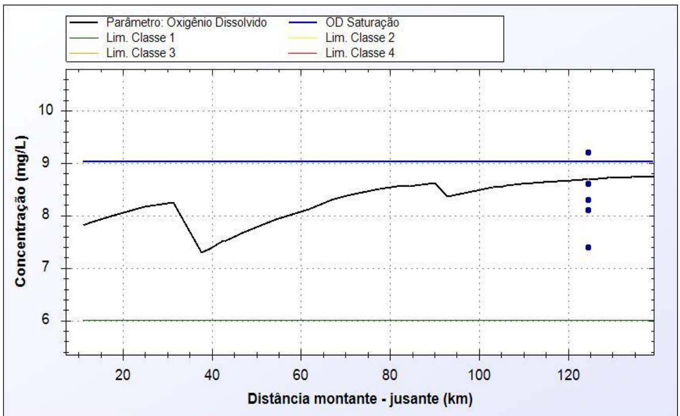
Figura 5.12 - Perfil de concentração ao longo do Rio Cotaxé: OD.
