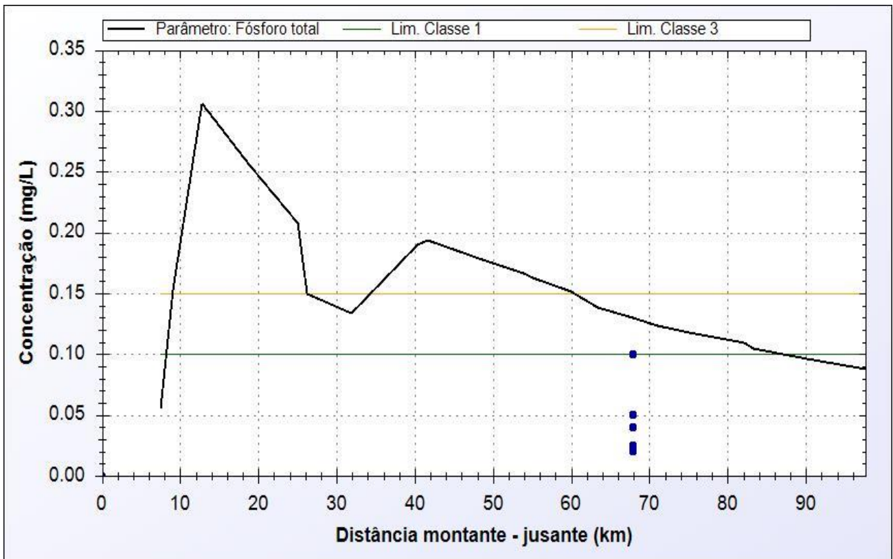
Figura 5.7 - Perfil de concentração ao longo do Rio Cricaré: fósforo total.
