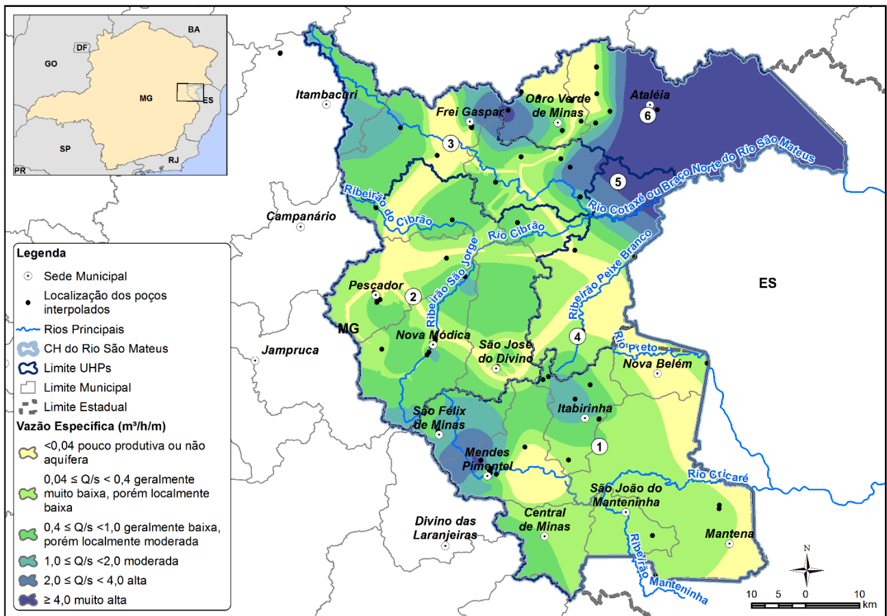
Figura 6.5 – Potencialidade dos aquíferos nas UHPs da Bacia Hidrográfica do Rio São Mateus
