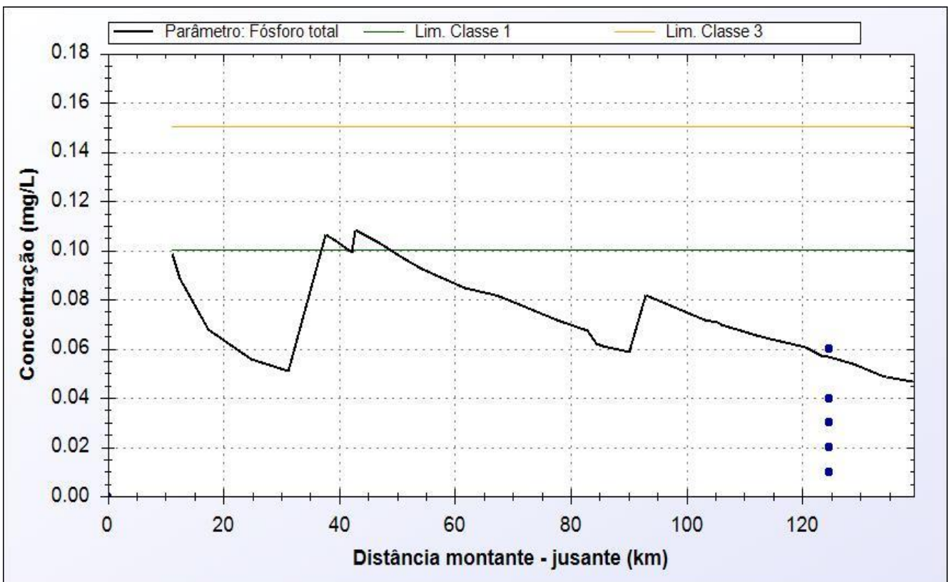
Figura 5.14 - Perfil de concentração ao longo do Rio Cotaxé: fósforo total.
