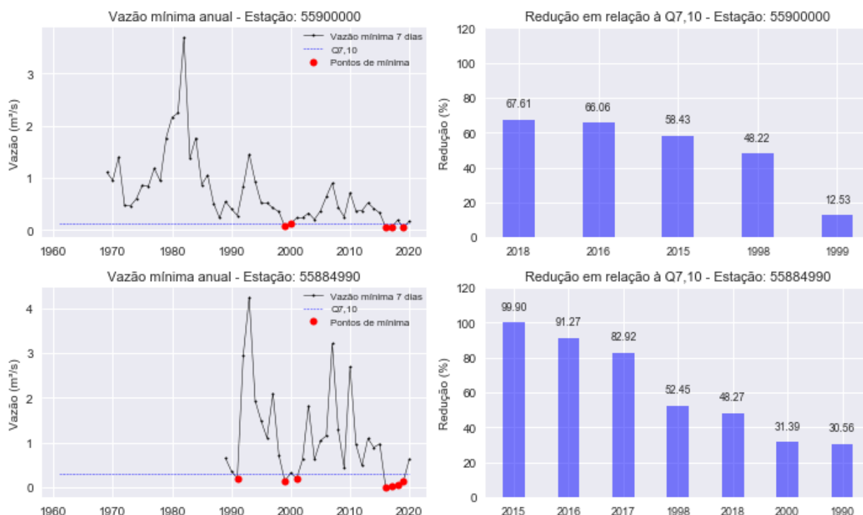
Figura 3.3 - Análise das séries de vazões mínimas anuais de sete dias de duração e comparativo com a Q_{7,10} nas estações fluviométricas da Bacia Hidrográfica do Rio São Mateus (Afluentes do Rio Cricaré).
