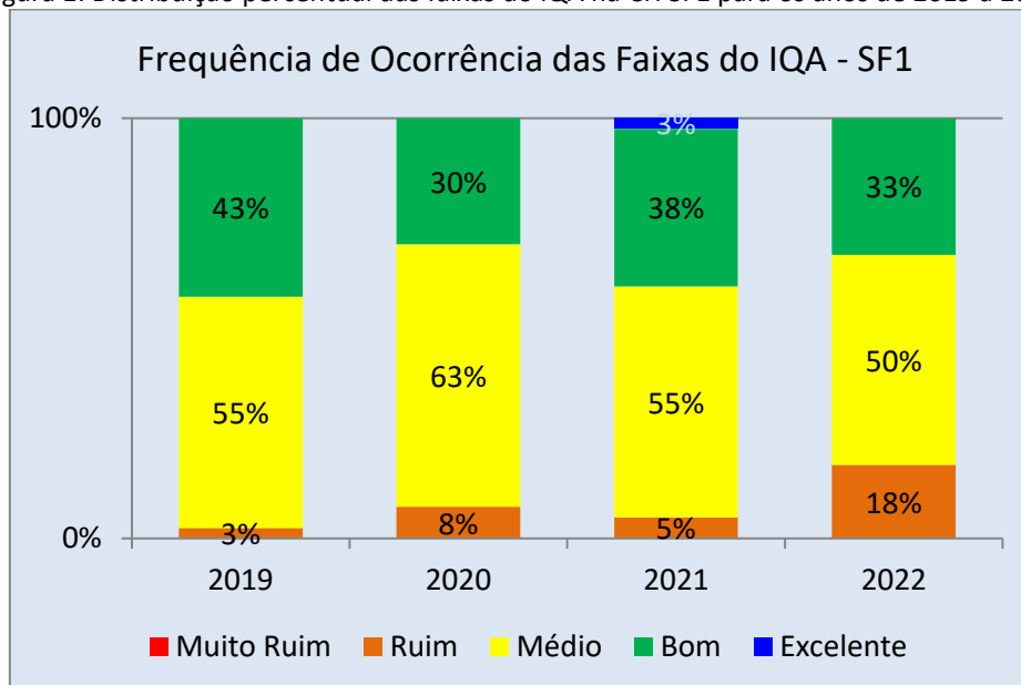
Figura 1: Distribuição percentual das faixas do IQA na CH SF1 para os anos de 2019 a 2022.
