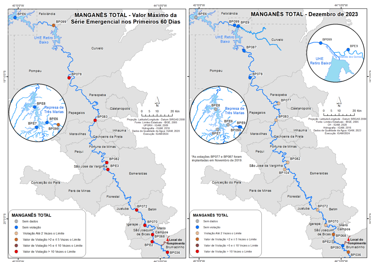
Figura 9 - Resultados de manganês total para cada estação de monitoramento nos primeiros 60 dias após o rompimento da B-I e os resultados do mês de dezembro 2023
