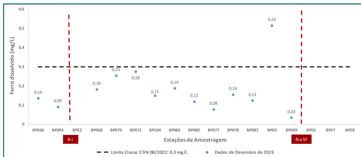
Figura 12 - Resultados de ferro dissolvido para dezembro de 2023
