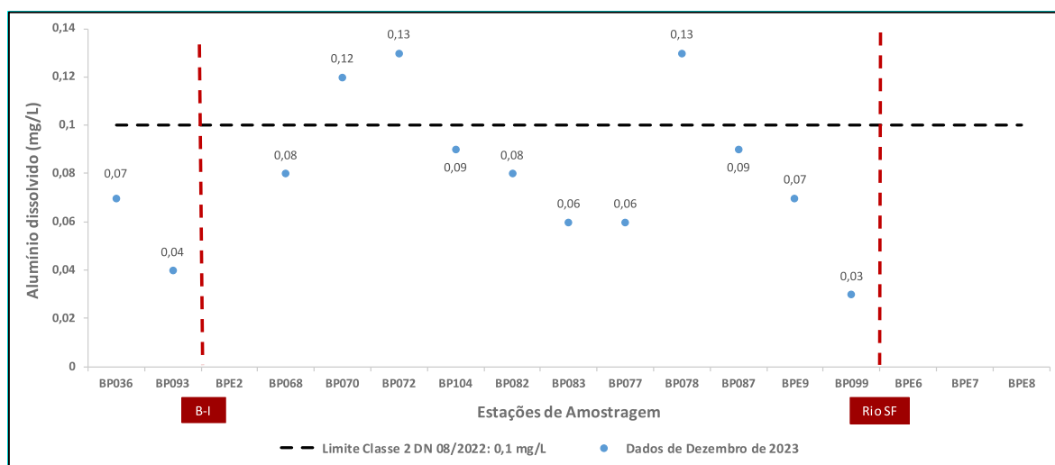
Figura 2 - Resultados de alumínio dissolvido para dezembro de 2023
