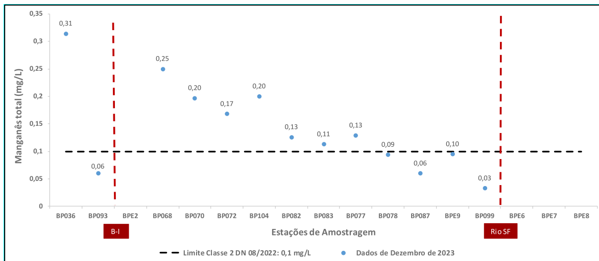
Figura 8 - Resultados de manganês total para dezembro de 2023
