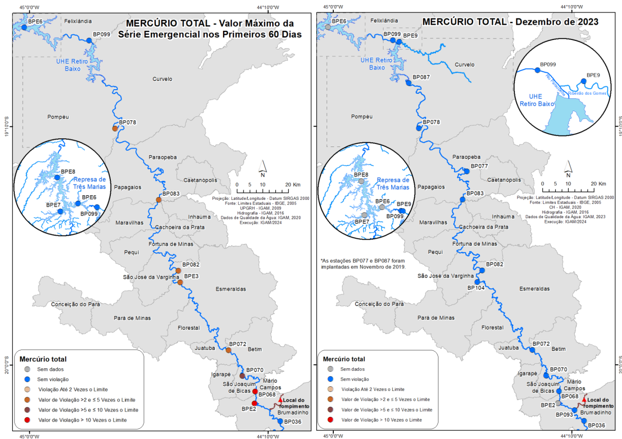
Figura 5 - Resultados dos valores máximos de mercúrio total para cada estação de monitoramento nos primeiros 60 dias após o rompimento da B-I e os resultados do mês de dezembro 2023
