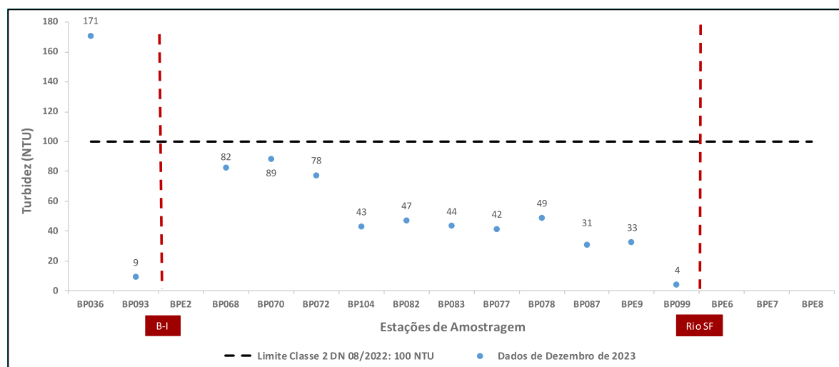
Figura 6 - Resultados de turbidez para dezembro de 2023
