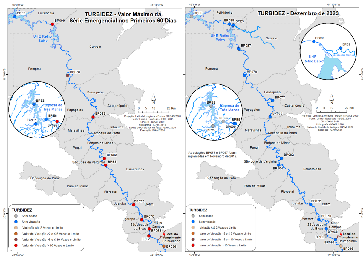
Figura 7 - Resultados dos valores máximos de turbidez para cada estação de monitoramento nos primeiros 60 dias após o rompimento da B-I e os resultados do mês de dezembro 2023
