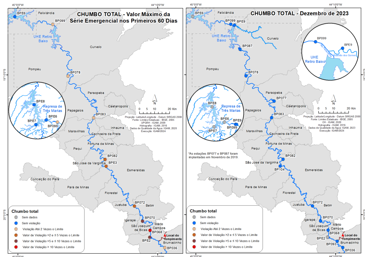
Figura 4 - Resultados dos valores máximos de chumbo total para cada estação de monitoramento nos primeiros 60 dias após o rompimento da B-I e os resultados do mês de dezembro 2023
