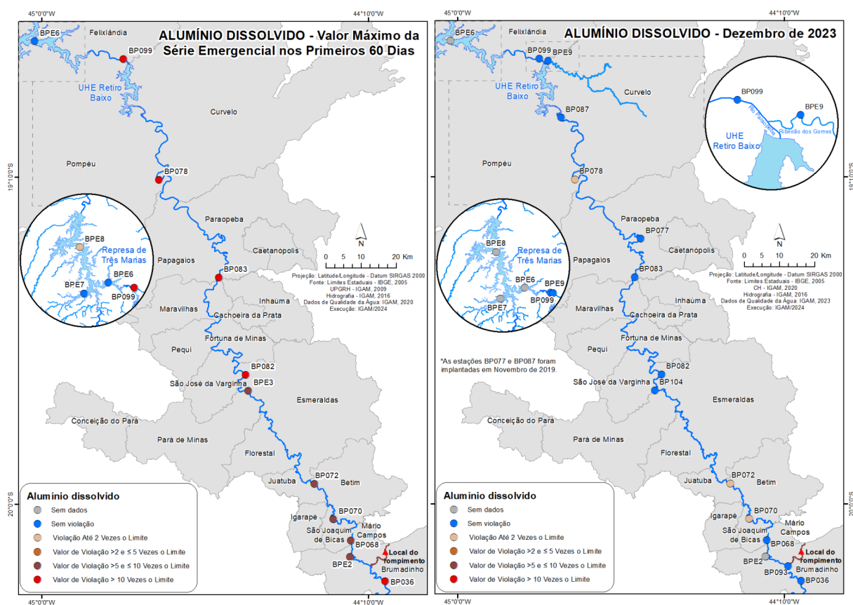
Figura 3 - Resultados dos valores máximos de alumínio dissolvido para cada estação de monitoramento nos primeiros 60 dias após o rompimento da B-I e os resultados do mês de dezembro 2023
