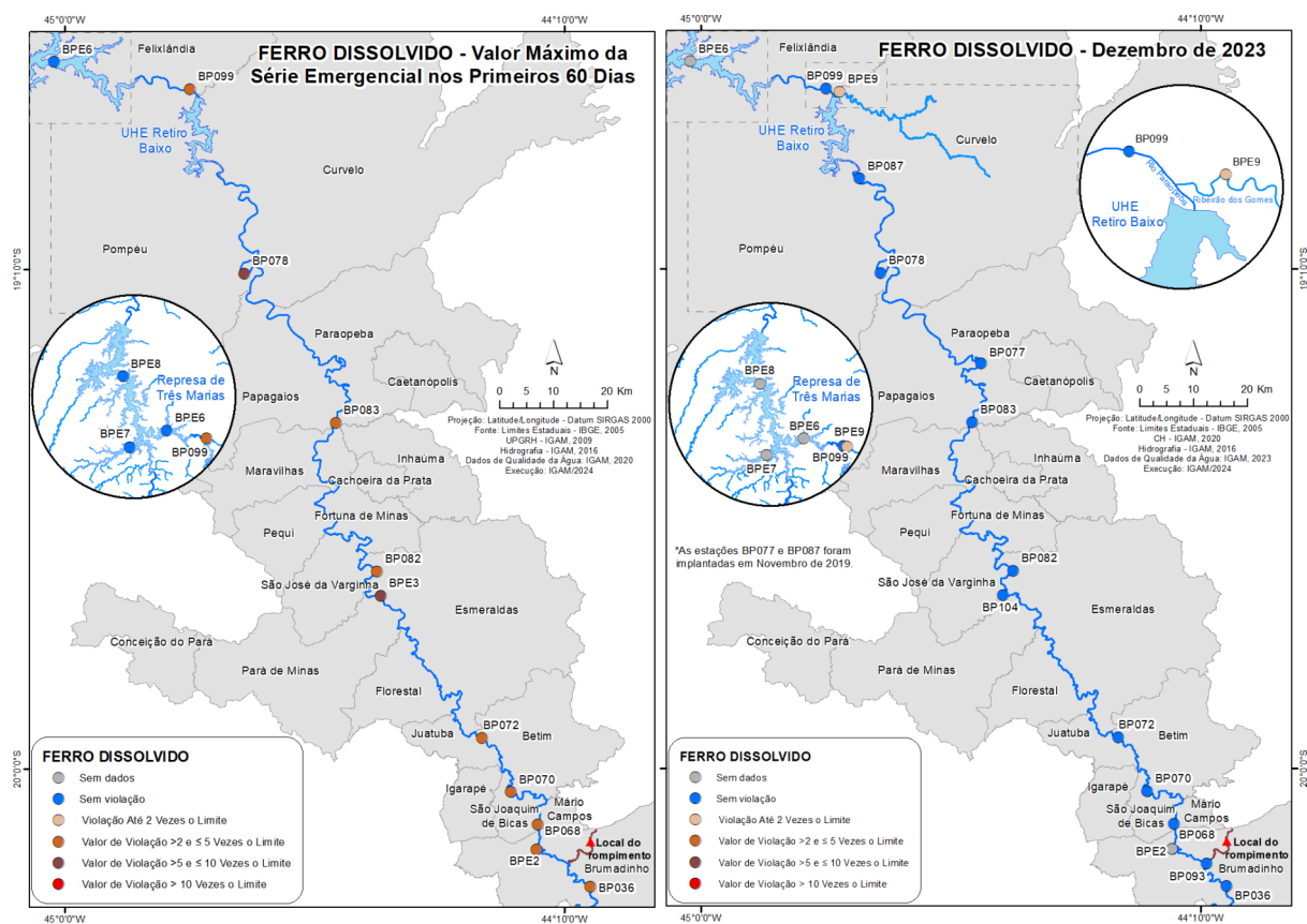
Figura 13 - Resultados dos valores máximos de ferro dissolvido para cada estação de monitoramento nos primeiros 60 dias após o rompimento da B-I e os resultados do mês de dezembro 2023
